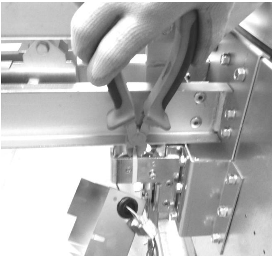
Rys. 41 Przycinanie opaski zaciskowej w celu odbezpieczenia zamka.
