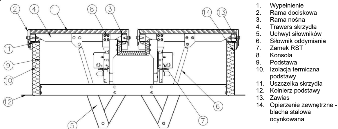
Rys. 1 Kłapa mcr PROLIGHT typu DVP - sterowanie.
