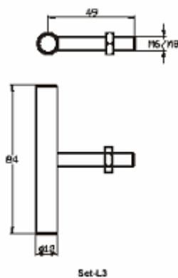
Rys. 21 Śruba 'T'.
