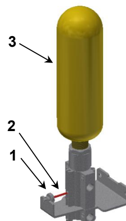
Rys. 30 Termowyzwalacz (na przykładzie TAVZ-4).
