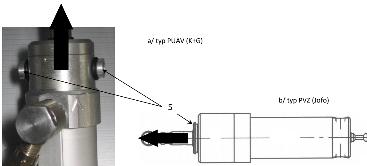
Rys. 32 Siłownik pneumatyczny – zwolnienie rygla.
