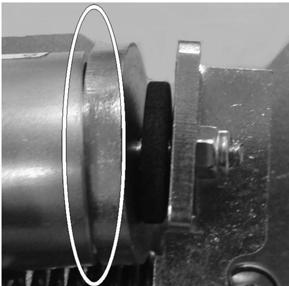
Rys. 44 Nieprawidłowo wyregulowana zwora elektromagnesu.
