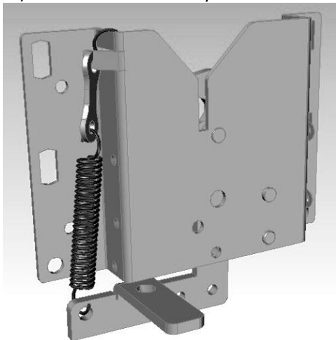
Rys. 38 Typy zamków dla sterowania mechanicznego.
