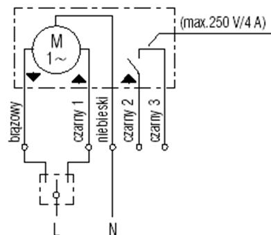
Rys. 37 Siłownik JMBB-500-300-LA.
