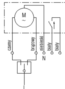
Rys. 36 Siłownik typu E-xxx-230.
