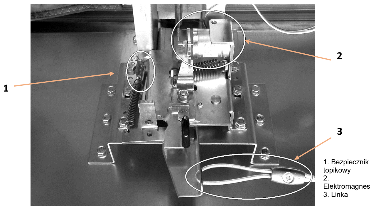
Rys. 39 Sposoby otwierania zamka.
