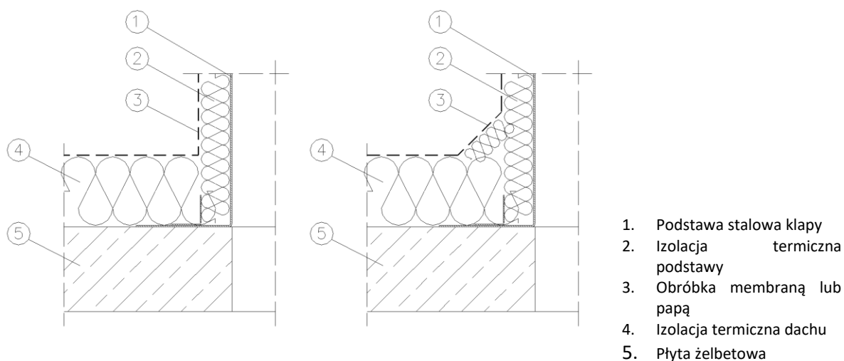
Rys. 7 Podstawa stalowa na płycie żelbetowej (a – obróbka membraną, b – obróbka papą).
