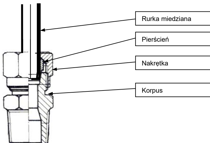
Rys. 25 Połączenie śrubunku z rurką miedzianą/stalową.
