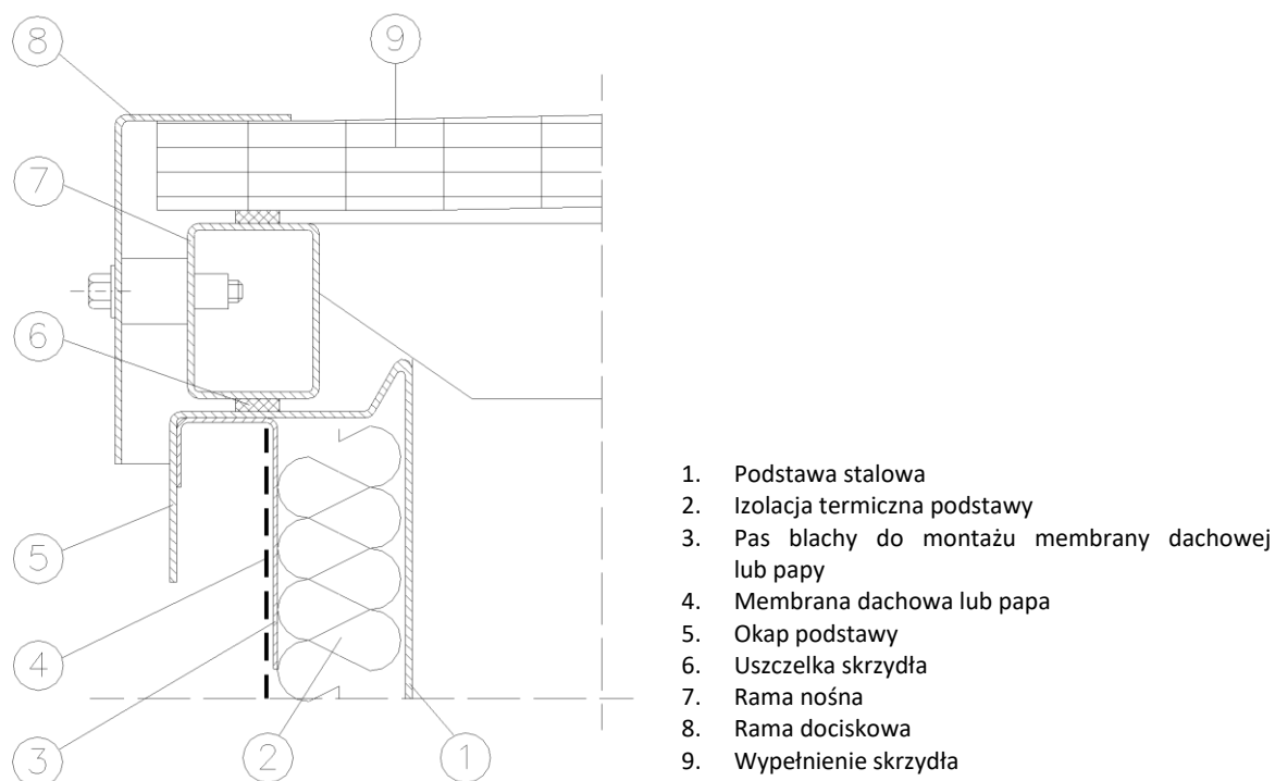
detal A
