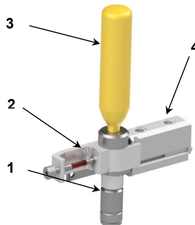
Rys. 29 Termowyzwalacz (na przykładzie TAVZ-3).
