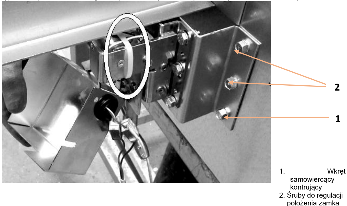
Rys. 40 Zamek zabezpieczony opaską zaciskową.
